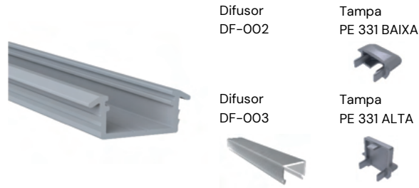
Perfil de Embutir – RM-331
