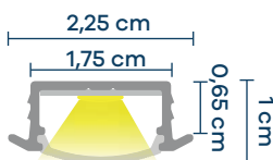
Difusor Baixo DF 002
