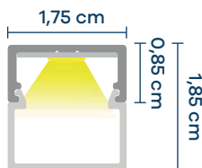
Difusor Alto DF 003
