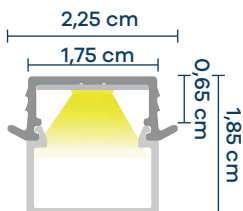
Difusor Alto DF 003
